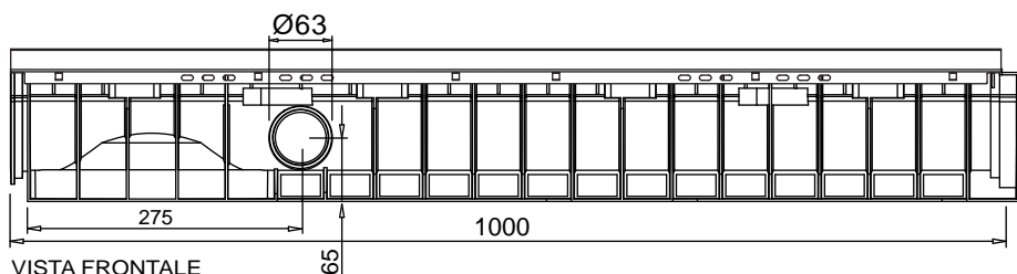
VISTA FRONTALE
