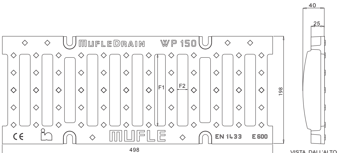
VISTA DALL'ALTO
