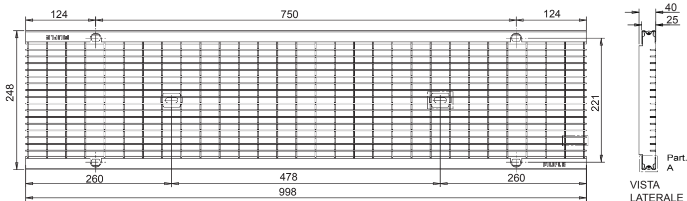
VISTA DALL'ALTO
