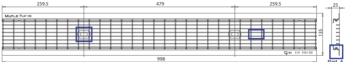
VISTA DALL'ALTO
