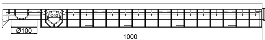
VISTA FRONTALE
