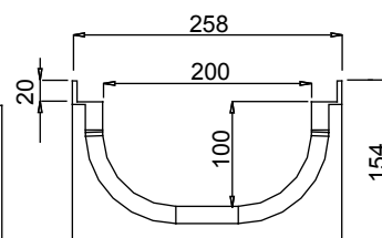
VISTA LATERALE
