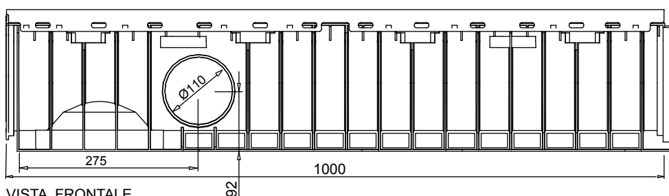
VISTA FRONTALE
